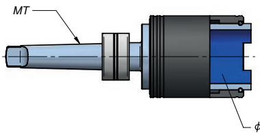
Gewindefutter - TC
