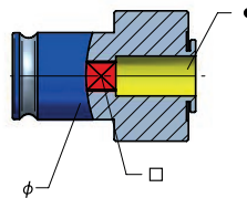
Gewindeadapter - TASC
