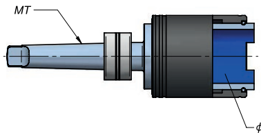
Gewindeschneidfutter - TC
