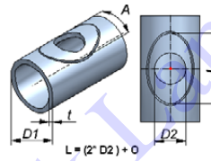
Sattel-Zuschnitt
