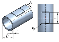
Rechteck-Ausschnitt
