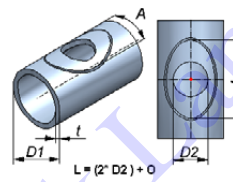
Sattel-Zuschnitt
