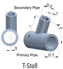
T-Stoß
