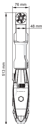
PRO 2 PB mit Elektromotor
