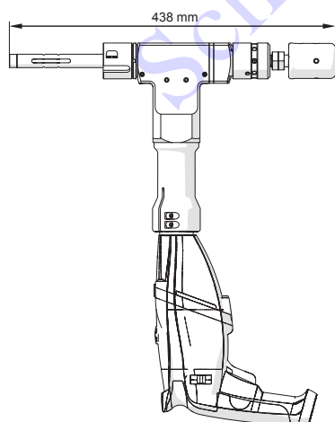
PRO 2 PB mit Elektromotor
