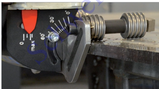
stufenlose Winkeleinstellung von 0° bis 60°
