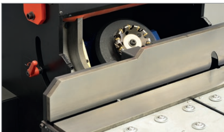
Einfacher Zugang zum Fräskopf und zu den Einsätzen
