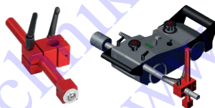
Rollenhalter PDT-0475-26-00-00-0
